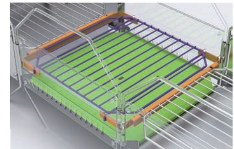
ジョイントパーツは焚火台本体フレームを連結し、中央部に組み込むことで3台分の焚火台として使用することが可能です。
